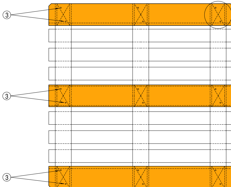
Unteransicht
